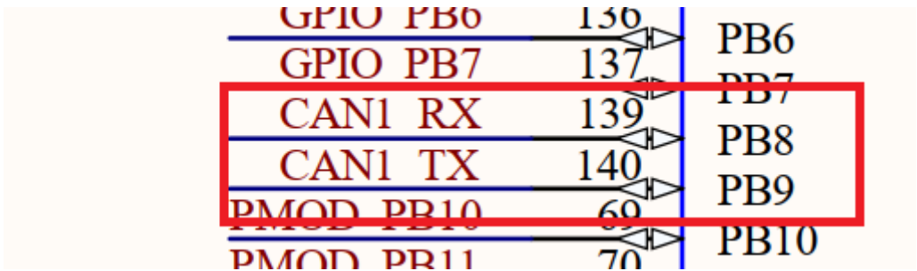
图 12.1: CAN 连接单片机引脚
