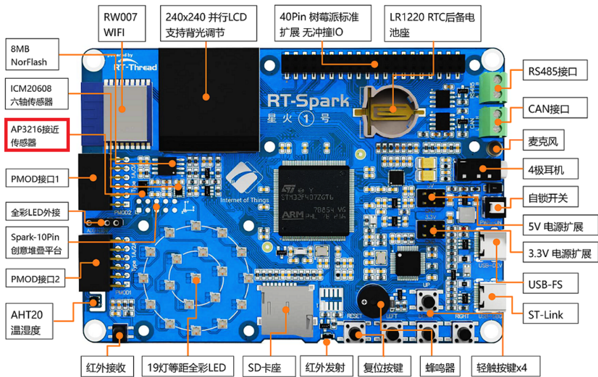
图 10.3: 接近与光强传感器位置
