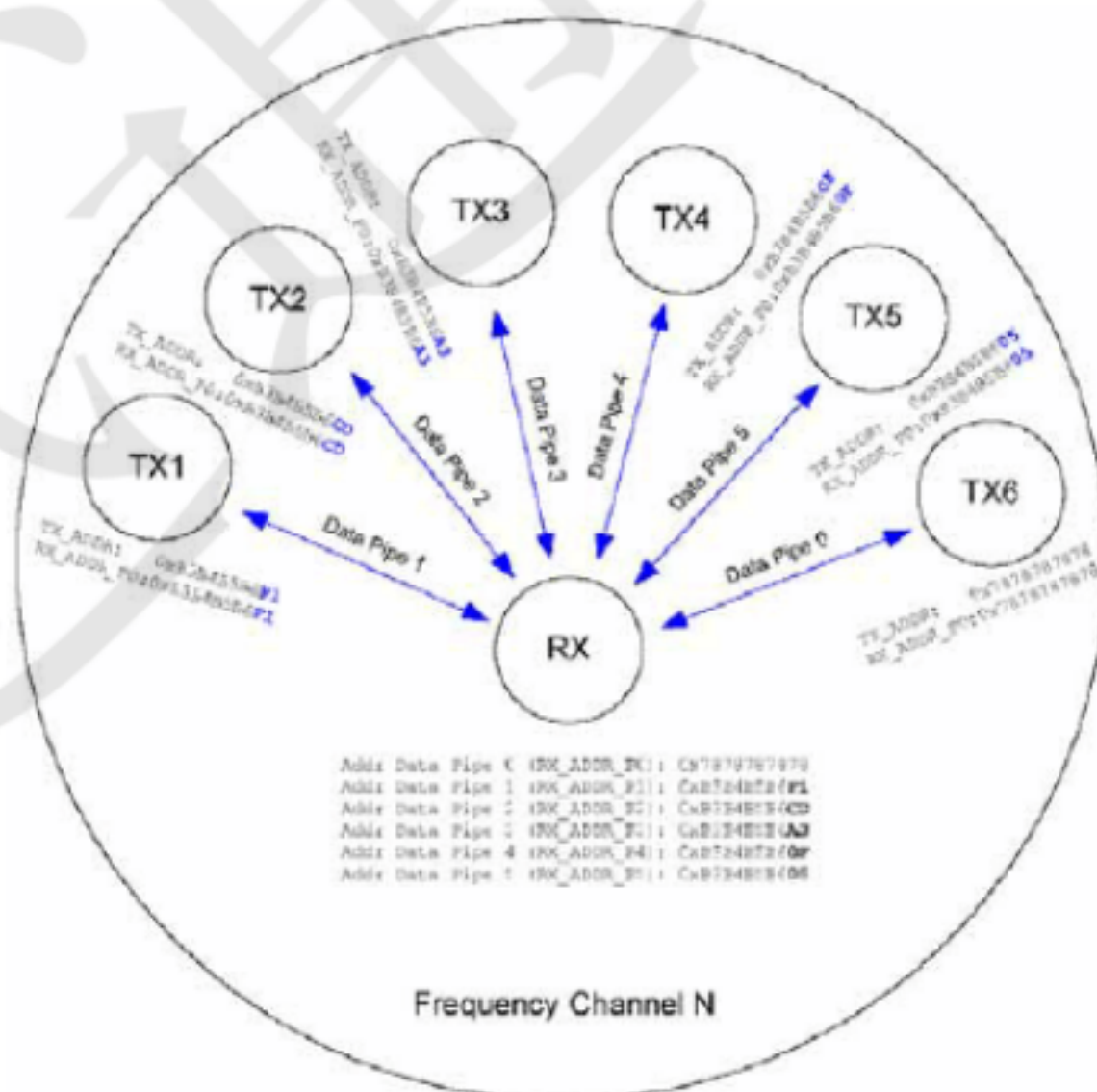
图 5、应答地址确定举例
