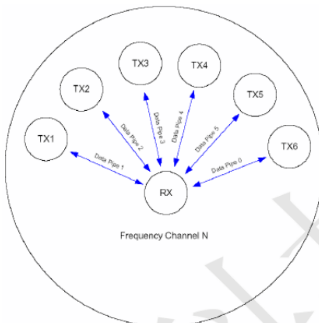
图 4、nRF24L01 在星形网络中的结构图
