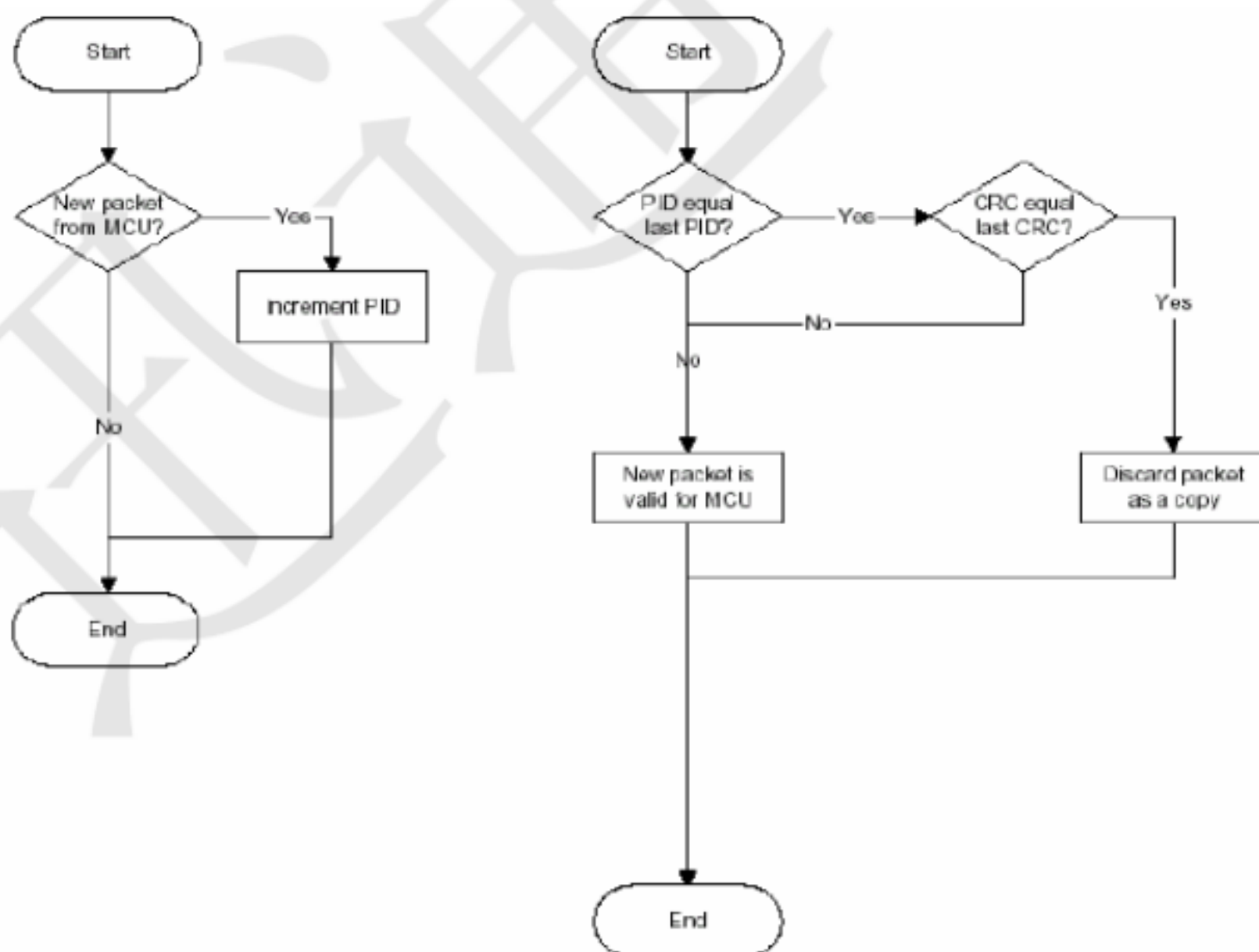
图 6、PID 值生成和检测
