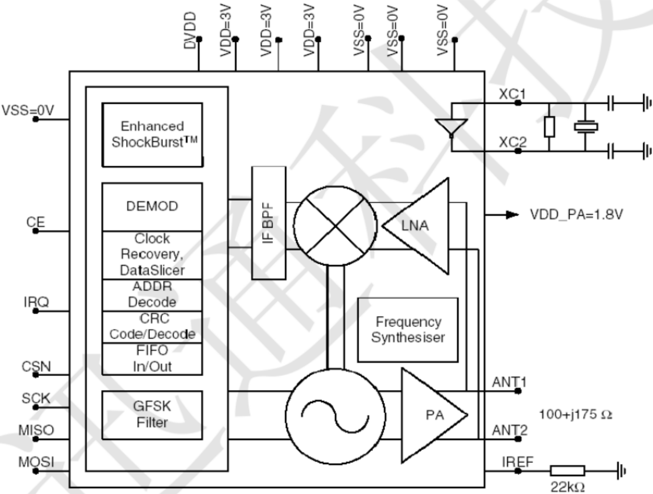
图 1 nRF24L01 及外部接口
