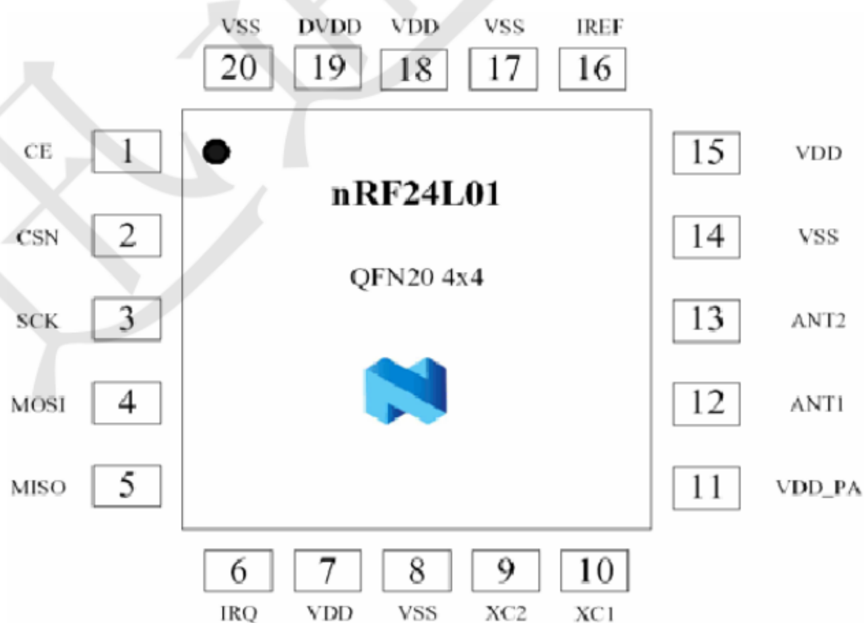
图 2、引脚封装
